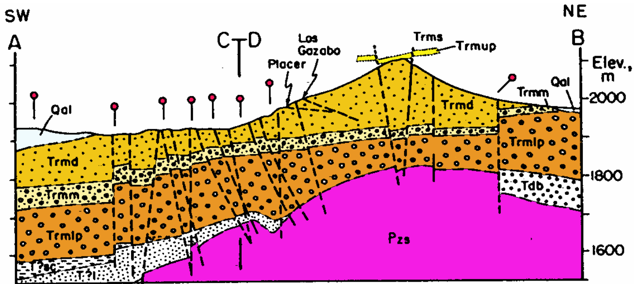
Fig. 3b Corte geológico vertical A-B del área de la mina Round Mountain {10}.
