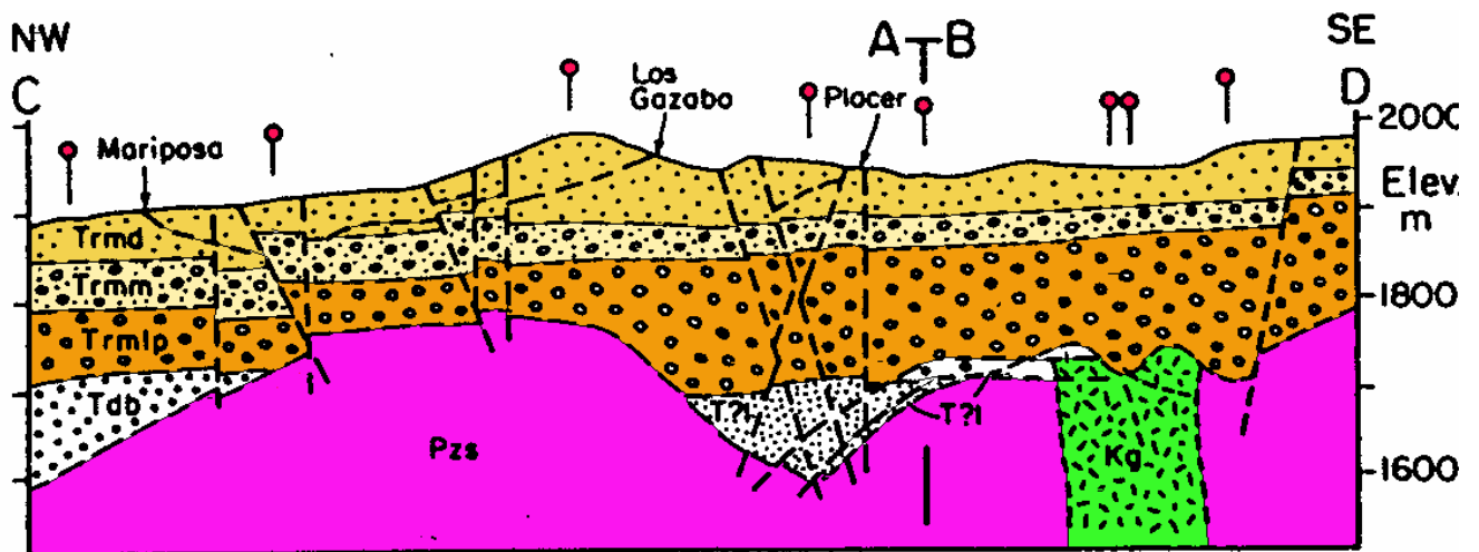
Fig. 3c Corte geológico vertical C-D del área de la mina Round Mountain {10}.
