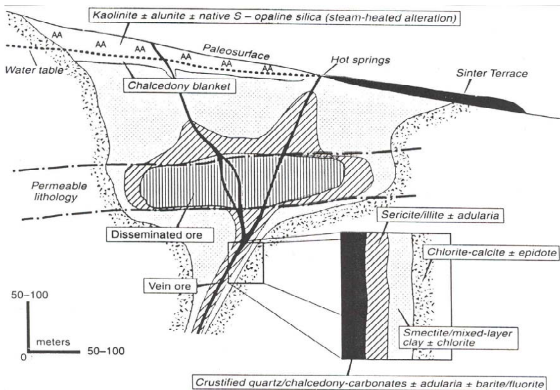
Fig. 5 Corte esquemático que generaliza los patrones de alteración en un sistema de baja sulfuración, mostrando las variaciones en profundidad, y típica alteración hidrotermal, incluyendo la distribución de sinter, capa de alteración argílica avanzada (AA), alteración por calentamiento con vapores, y silicificación asociada con el nivel freático (según Buchanan, 1981 y Sillitoe, 1993). Las variaciones geológicas de los diversos yacimientos presentan múltiples desviaciones de esta generalización {3b}.
